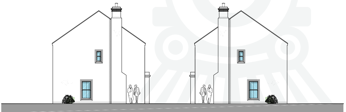
FLANK ELEVATION
