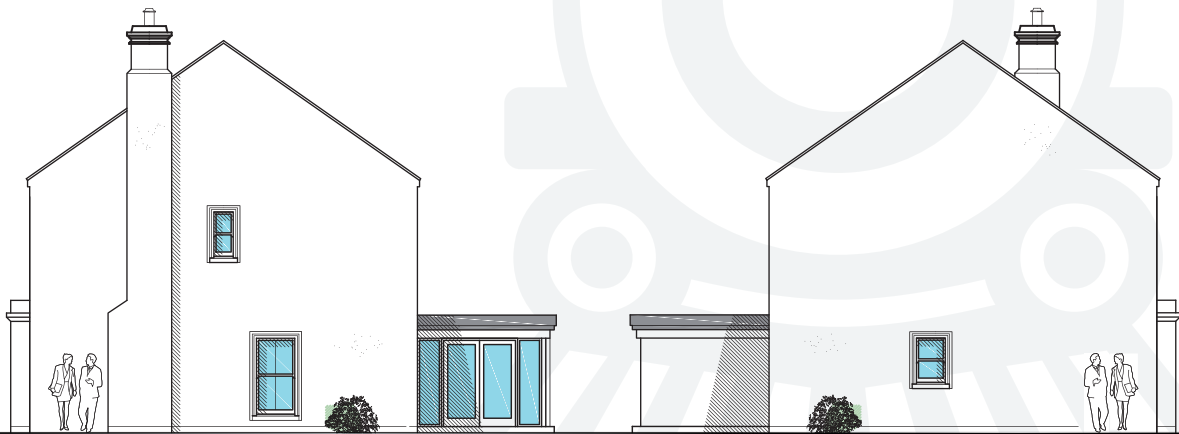
FLANK ELEVATION
